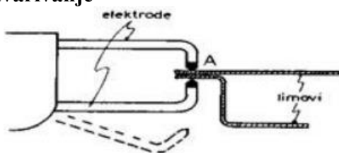
Sl. 16. Tačkasto zavarivanje
