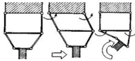
Sl. 31. Pasivno popuštanje
