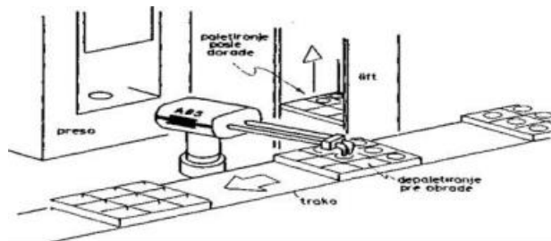
SI. 8. Transport palete pokretnom trakom
