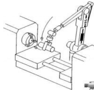
Sl.13. Robot opslužuje strug
