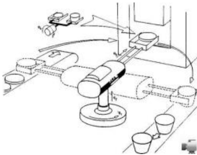
Sl. 12. Opsluživanje prese
