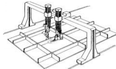
Sl. 21. Dvoručni portalni robot za zavarivanje
